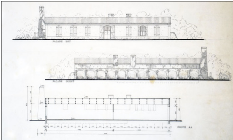
• Relevé de l'habitation Desglaireaux à Quartier-Morin (Projet Route 2004 • Marie Brémaud, Architecte, 1996)
