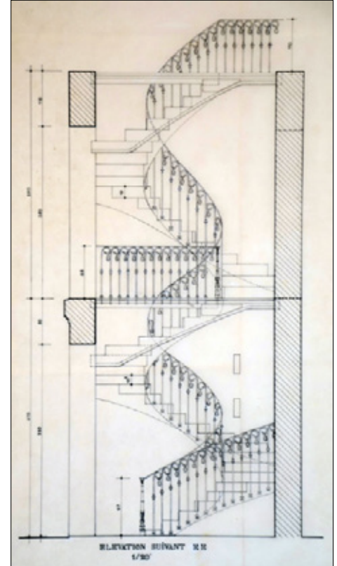
• Relevé de l'escalier de la maison Firmin au Cap-Haïtien (Projet Route 2004 • Marie Brémaud, Architecte, 1996),
